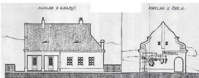
Z projektu výpravnej budovy v Budkovciach, 1924
